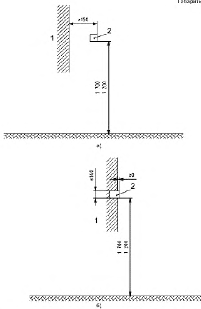
Рисунок 4 — Расположение барьера при хранении машины
