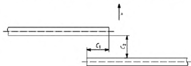
а) Расстояние между двумя частями защитного приспособления
