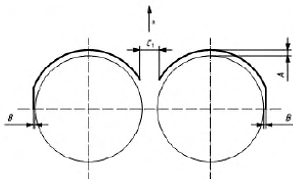
г) Защитное приспособление, огибающее ротор
