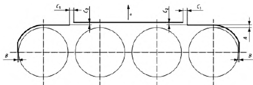
е) Несколько роторов, расположенных на одной линии
