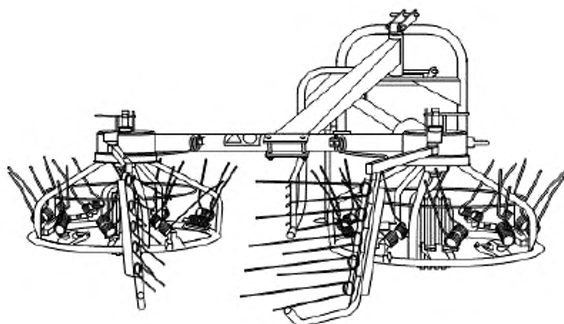
Рисунок А.5 — Ротационные барабанные грабли
