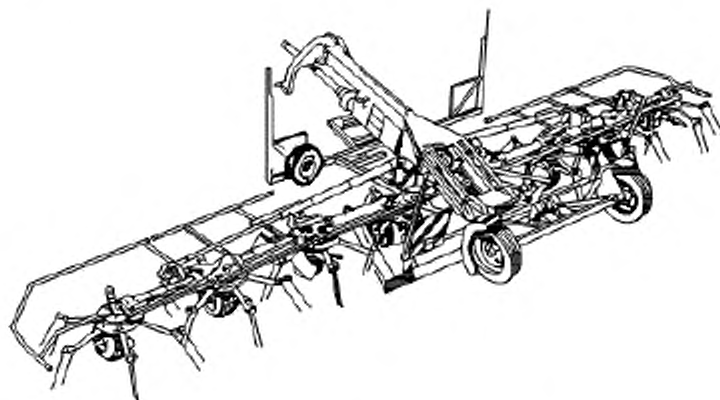
Рисунок А.1 — Полунавесная сеноворошилка
